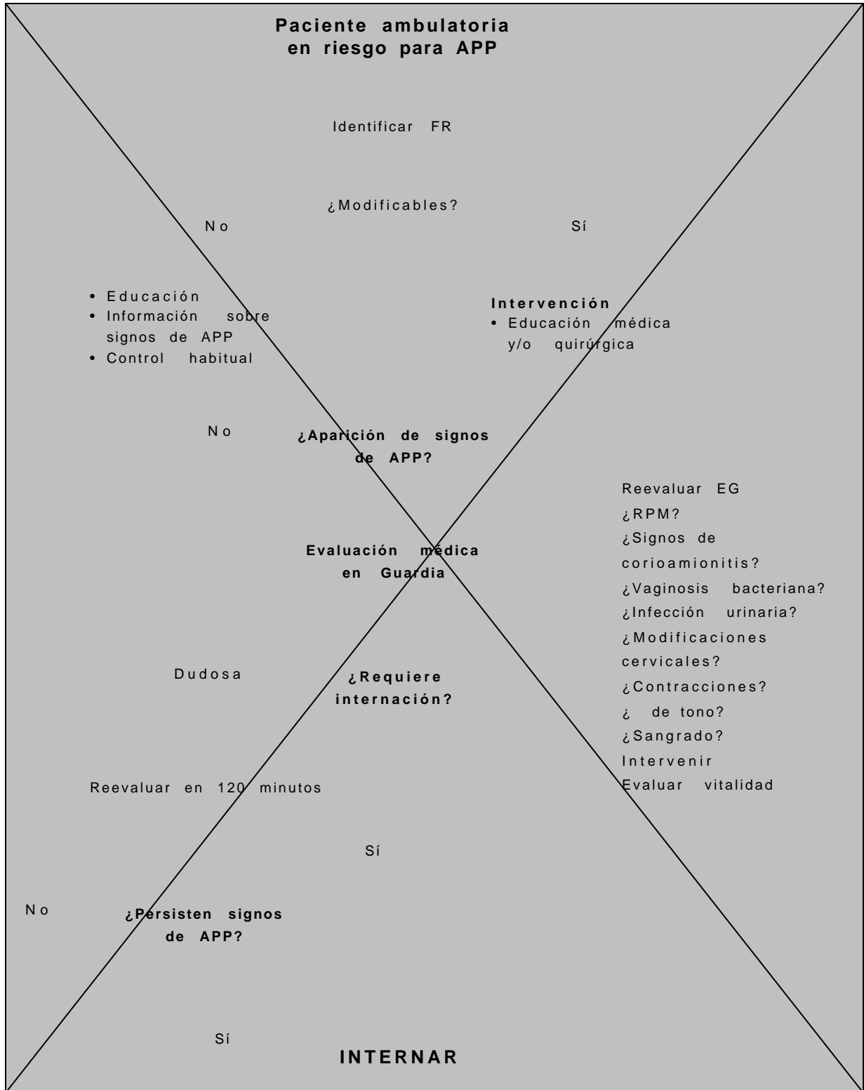
Figura 1: Algoritmo
