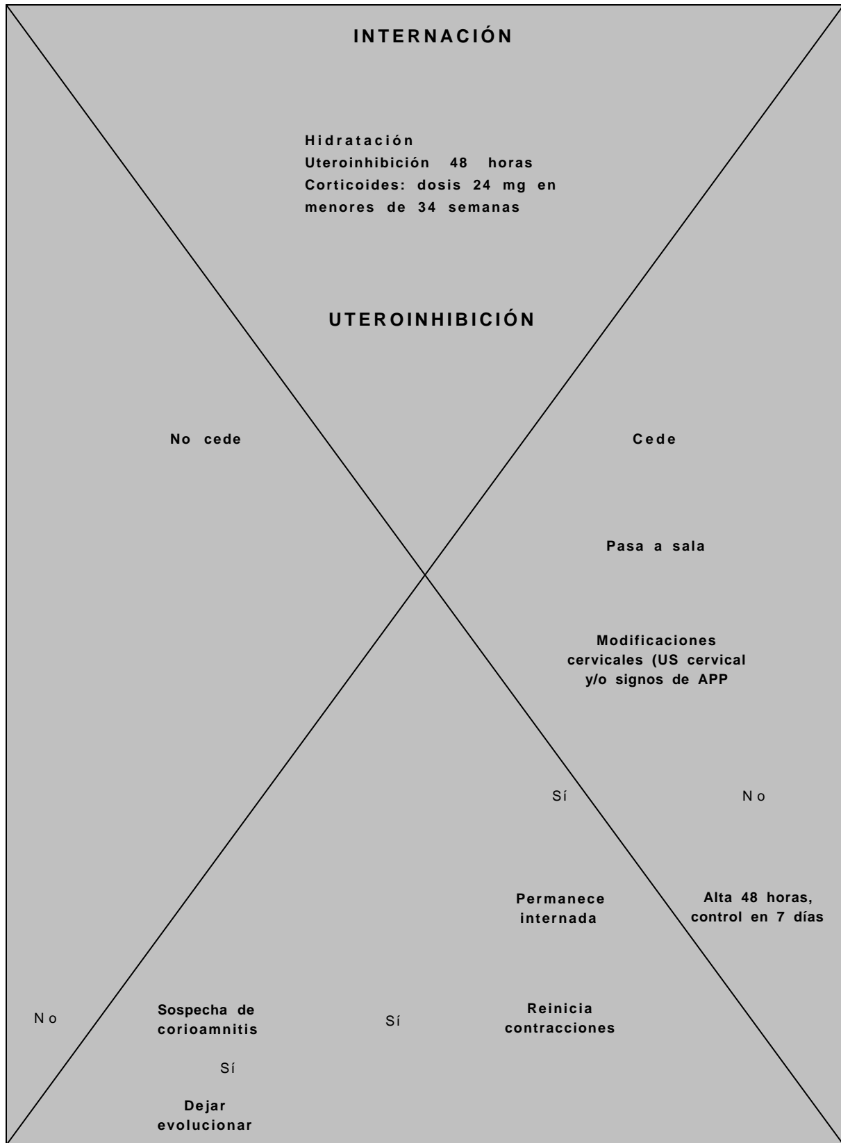
Figura 2: Algoritmo
